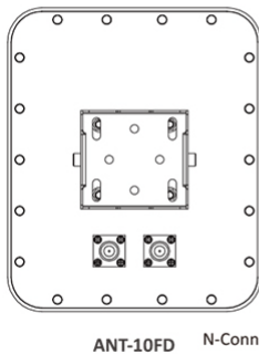
2.4Ghz Antenna
